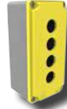
BT4-3001-0017 80mm x 170mm x 73mm 4'lü Alümi. Buat (IP67) Kutu Adedi: 1
